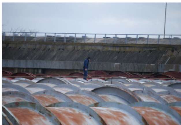
Рис. 1/5 Расходомеры-счетчики IPKA, установленные на Главной насосной станции подачи воды в магистральный канал. Диаметр труб 3600 мм
