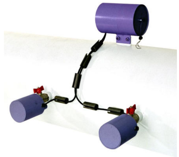
Рис. 1/2 Ультразвуковой расходомер-счетчик ИРКА.
